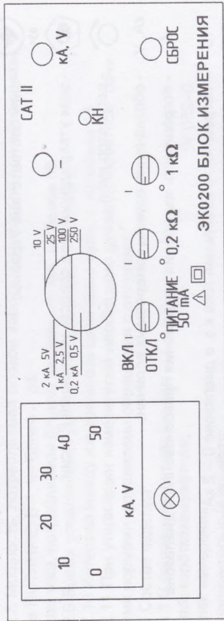
Рисунок 1.1 - Передняя панель блока измерения
